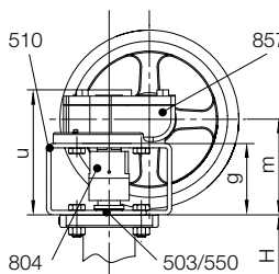
Aufbau Schneckengetriebe bei Klappe mit Sicherheitsstopfbuchse
