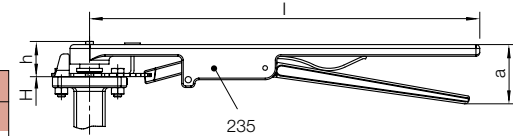
(Handhebel DN 65, 125, 450-750 für Klappen mit PFA-ummanteltem Teller siehe S. 8)
